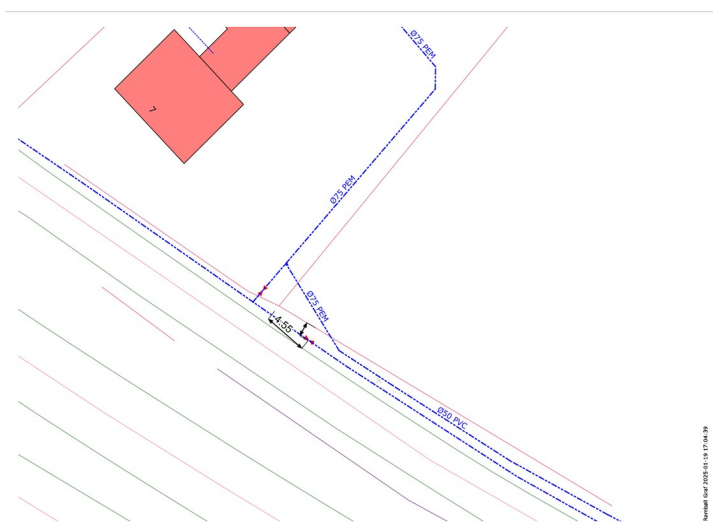
vandtårnet udsnitning af ventil på forsyningsledning til andelsnaverne på vandtårnet
